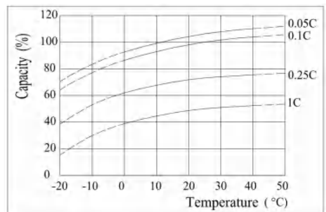
温度与容量关系曲线
